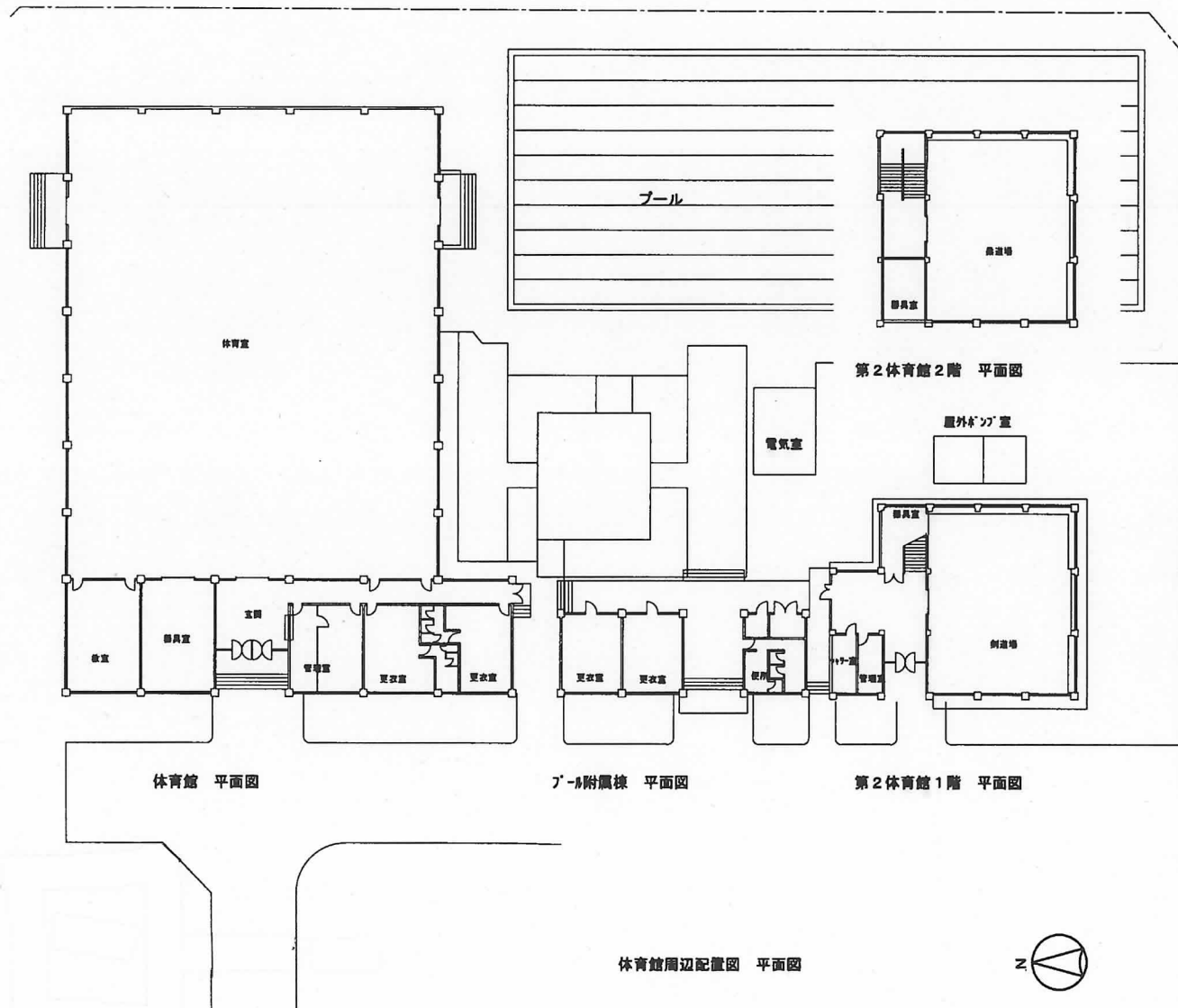
体育館・第2体育館・プール平面図
